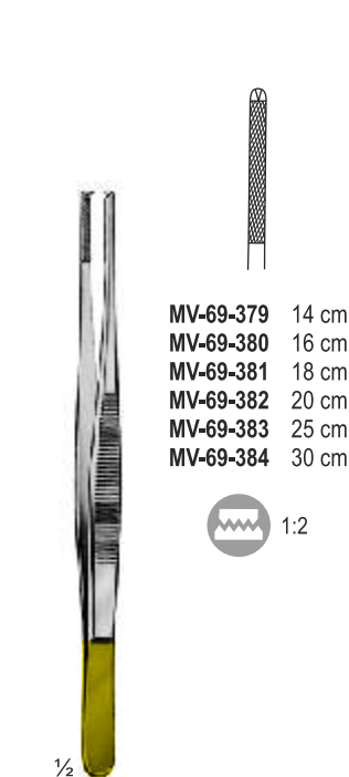
Oehler MV-69-379 - MV-69-384 14 cm
